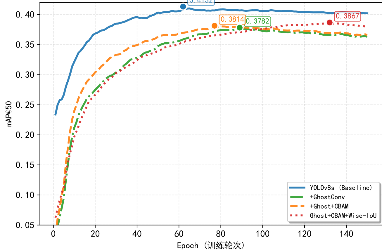
mAP@50 性能对比
