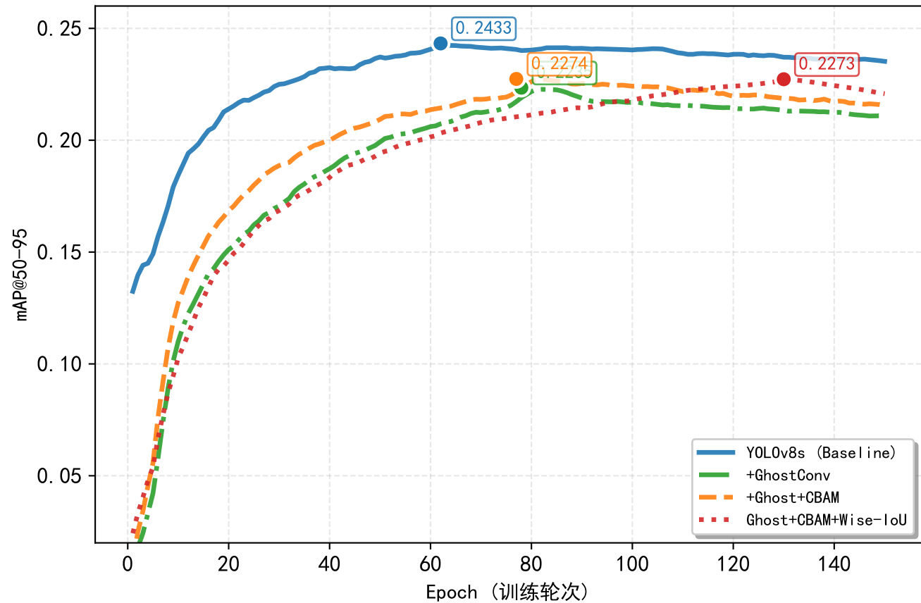
mAP@50-95 性能对比
